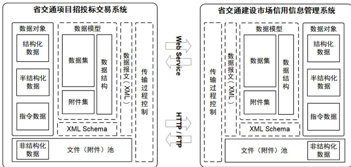
对接总体框架示意图
